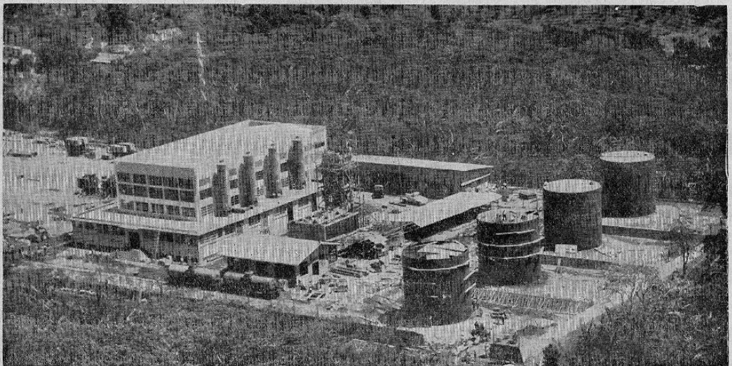
Vista aérea del conjunto que constituye la Central Diesel Eléctrica de Colima. A la izquierda se ve el edificio de casa de máquinas con sus grandes chimeneas, otras obras al centro, y a la derecha los tanques para combustible, con capacidad para 150 mil galones cada uno.
